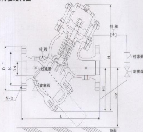
产品外观及内在结构图
